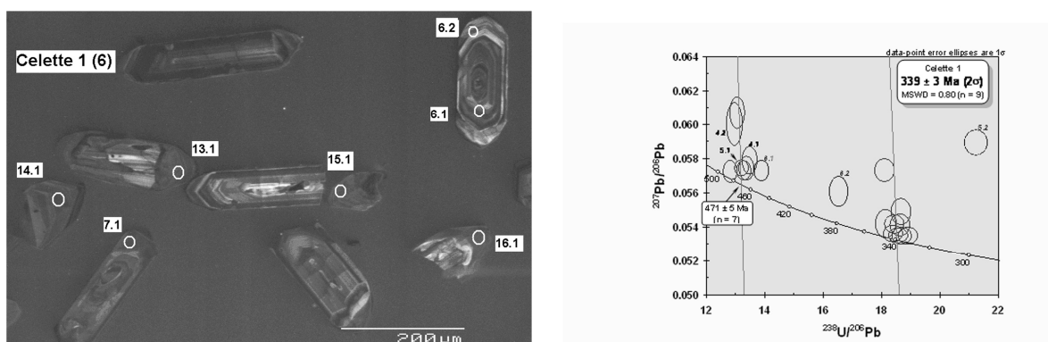
Figure 109 : photos des zircons en cathodoluminescence et diagramme Concordia pour la diatexite de la Cellette
