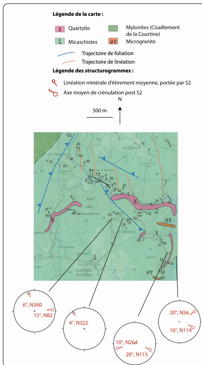
Figure 147 : carte géologique et structurale des micaschistes du Chavanon sur la feuille Ussel. Fond topographique IGN
