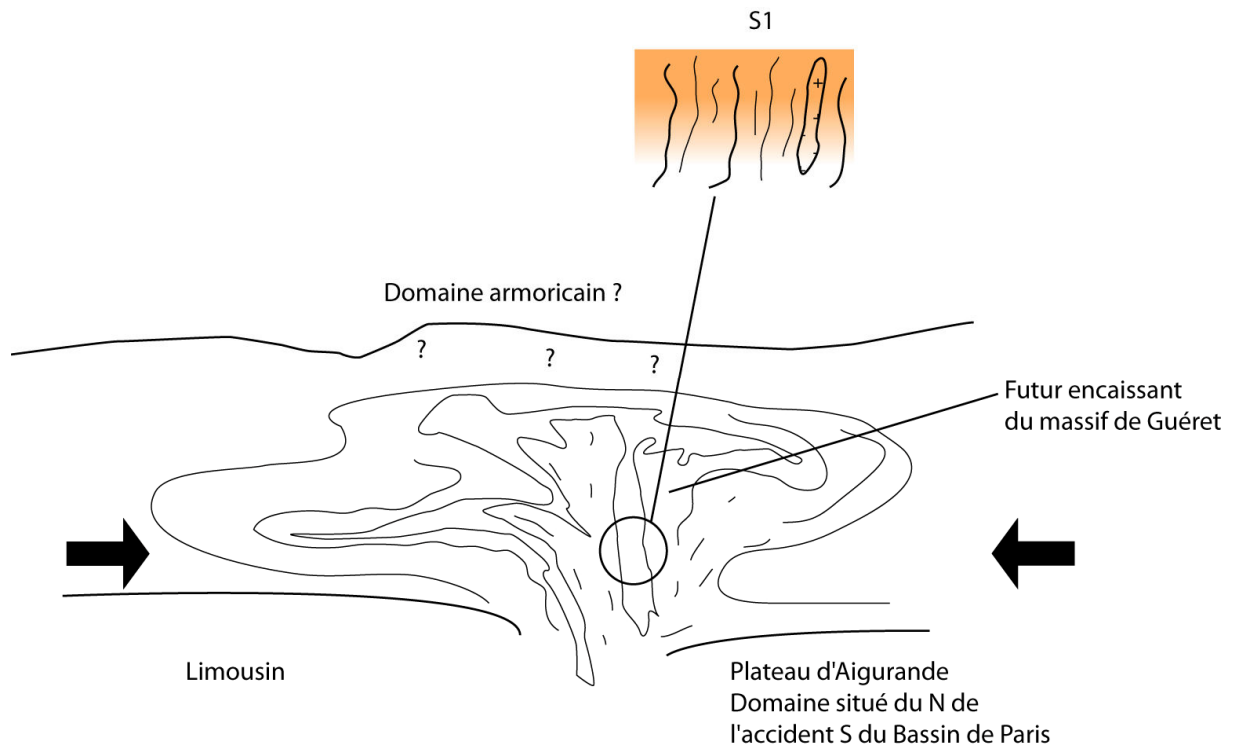
Figure 178 : dôme extrusif à cœur caractérisé par une foliation métatectique fortement pentée
