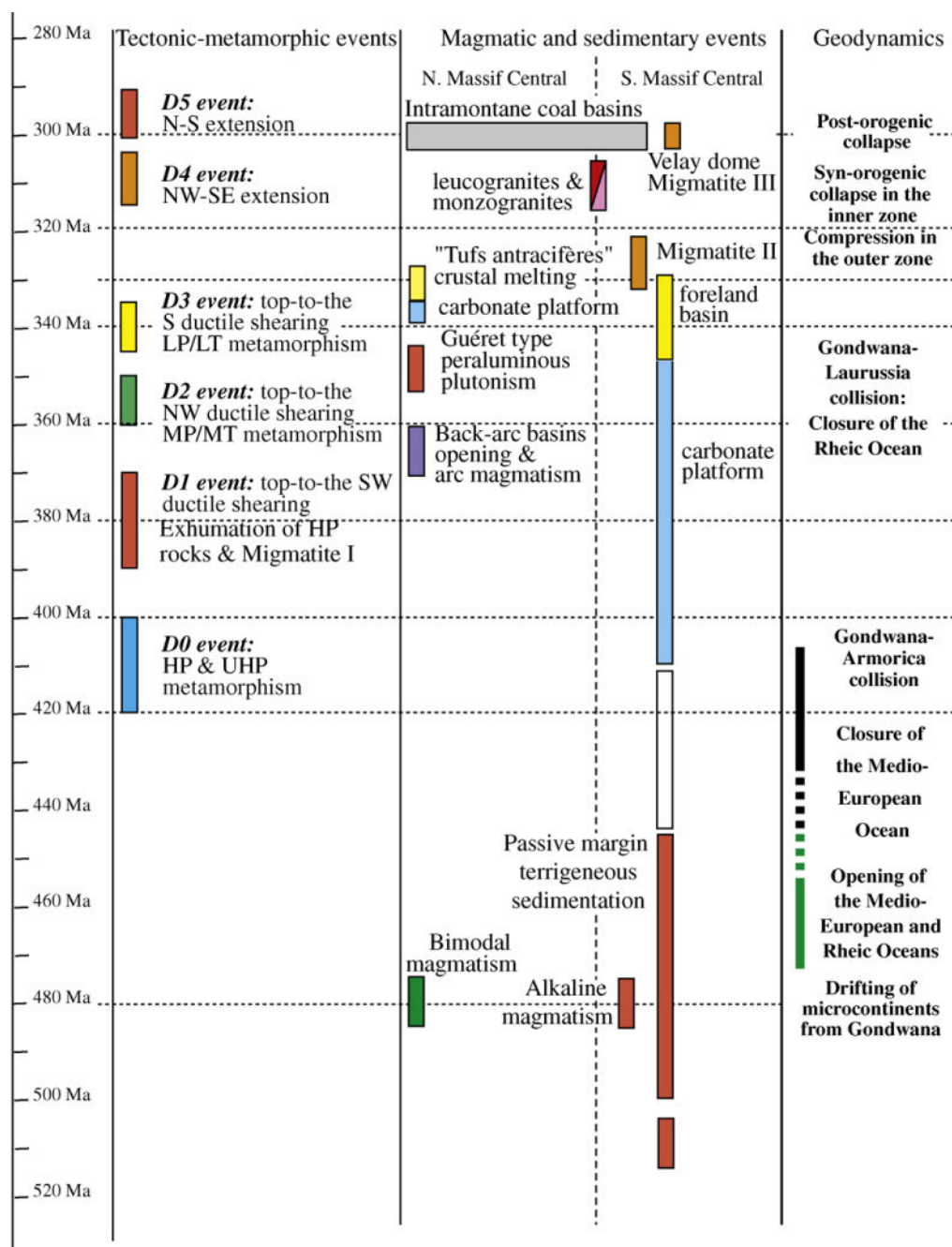
Figure 29 : tableau synoptique des événements tectono-métamorphiques, magmatiques et sédimentaires du Massif Central (Faure et al., 2009)
