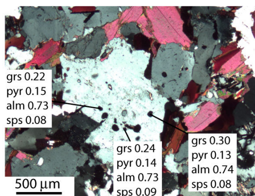
Figure 65 : inclusions de grenat dans les gneiss gris du Chavanon et analyses microsonde représentatives
