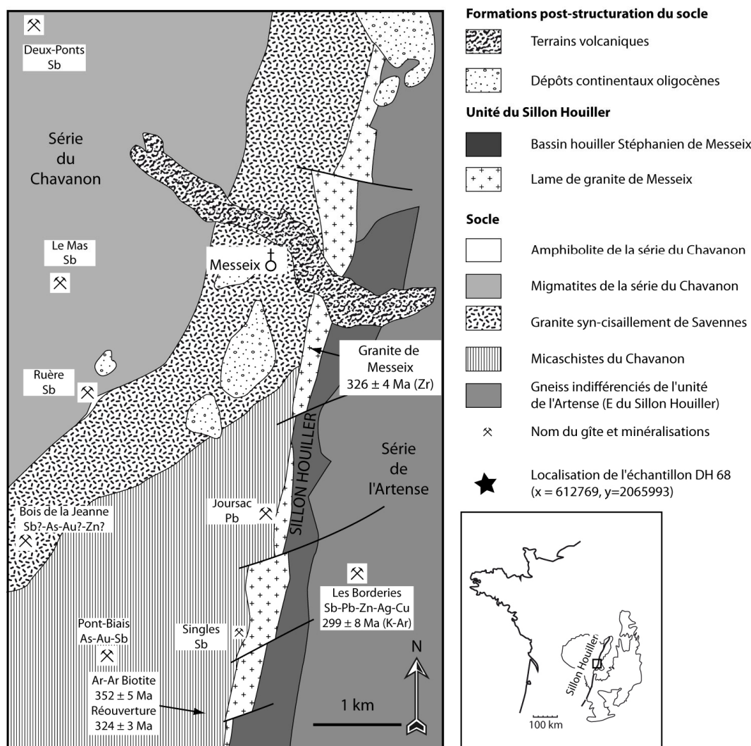
Figure 117 : localisation des minéralisations dans le cadre de la série du Chavanon et du Sillon Houiller
