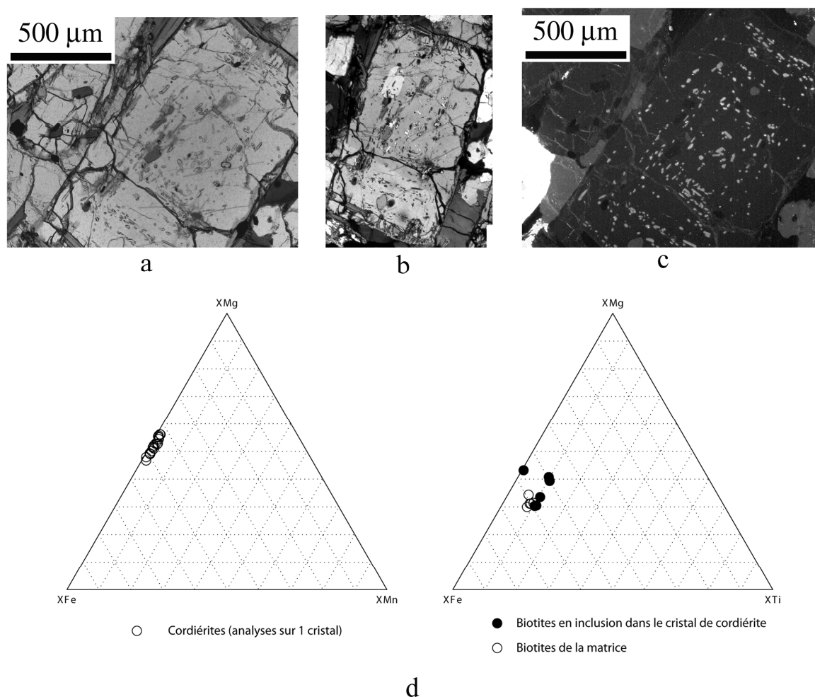
Figure 82 : photographies au microscope optique (a : LPNA, b : LPA) et en cathodoluminescence (c) d'un monocrystal de cordiérite riche en inclusions ; d : analyses chimiques sur le cristal et sur les biotites qu'il contient en inclusions
