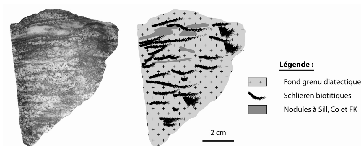
Figure 73 : nodules à sillimanite, cordiérite et FK dans les gneiss gris du Chavanon
