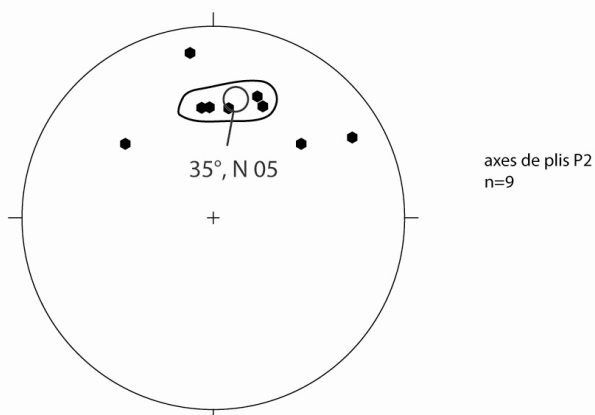
Figure 138 : plis P2 synfoliaux dans les gneiss de la série de la Sioule, reprenant une foliation S1 métatectique
