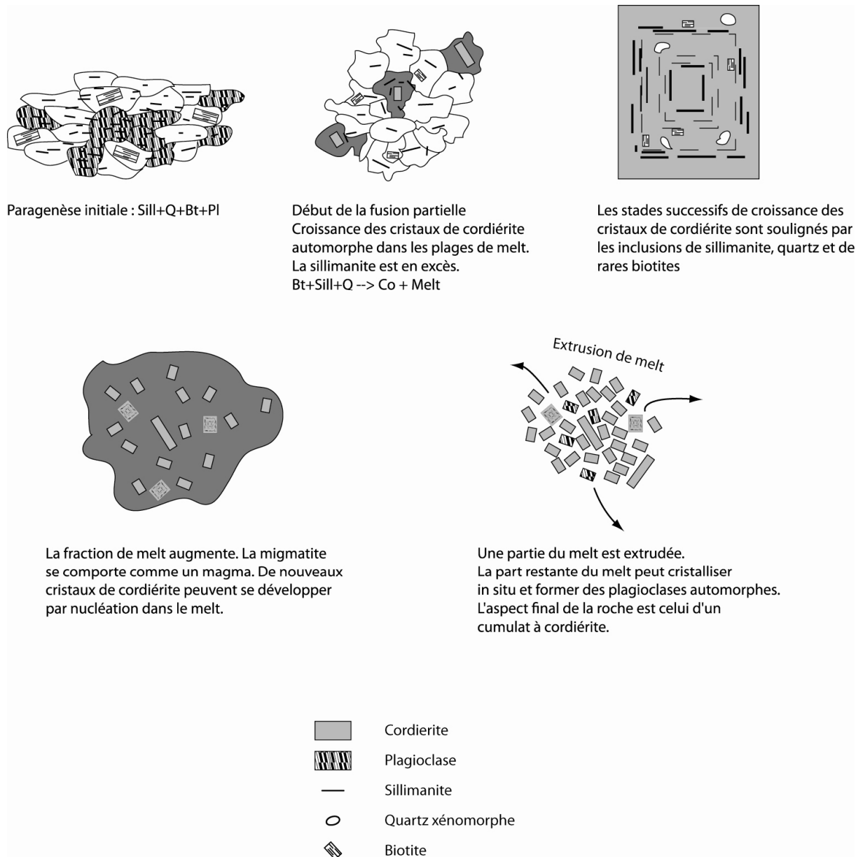
Figure 85 : modèle de formation des cordiérîtites
