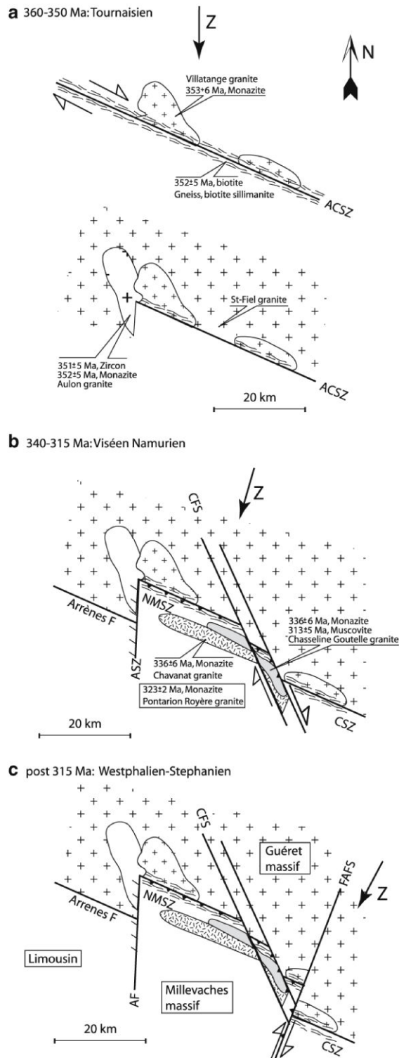
Figure 24 : évolution au Carbonifère (360-300 Ma) de la zone de cisaillement du nord-Millevaches-la-Courtine (Cartannaz et al., 2007)
