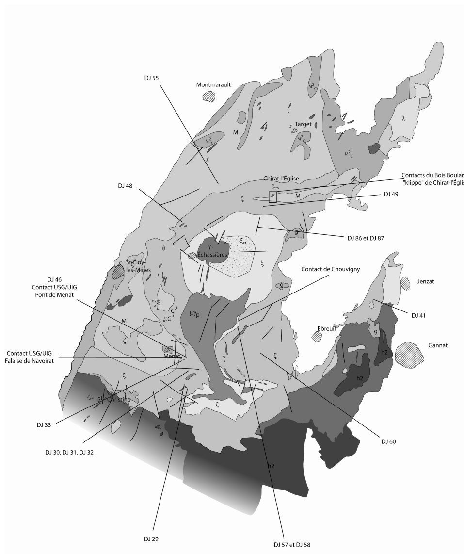
Figure 135 : carte de localisation des affleurements et secteurs décrits dans l'étude structurale de la série de la Sioule
