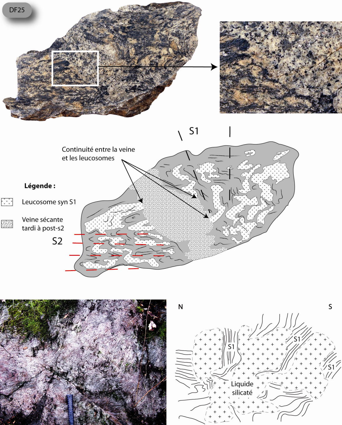
Figure 133 : migmatites polyphasées du sommet de la série du Chavanon, affleurement DF 25. La S1 peut être complètement démembrée par l'anatexie
