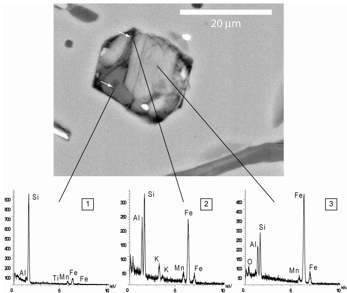
Figure 48 : étude au MEB et spectre EDS d'une inclusion polyphasée d'un grenat, représentant probablement une inclusion de type « nanogranite »
