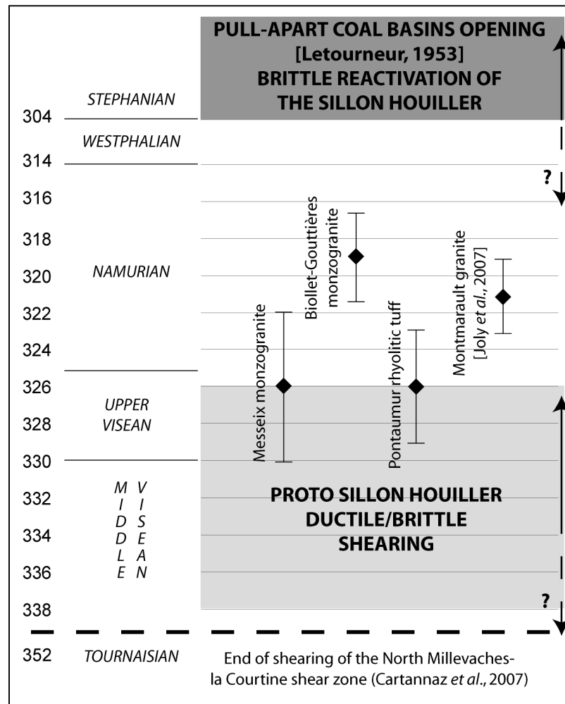
Figure 12 : Synthesis of tectonical and magmatic activity along the Sillon Houiller. Figure 12 : Synthèse des événements tectoniques et magmatiques le long du Sillon Houiller
