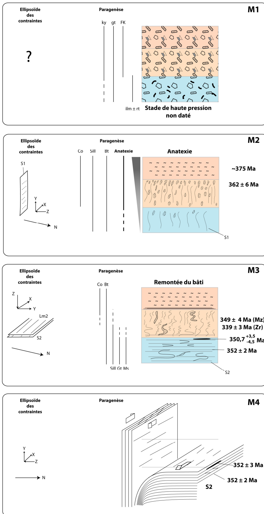
Figure 175 : synthèse conceptuelle de la succession des déformations et des métamorphismes associés
