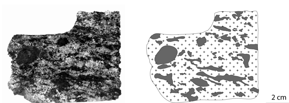
Stade 3 : les restites forment des nodules, plus ou moins allongés, selon la déformation subie par la roche.
