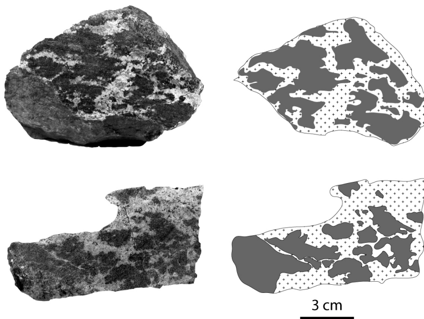
Stade 2 : la fusion partielle continue et individualise des domaines de gneiss hypercordiéritique. Plus le taux de fusion est élevé, plus la roche est riche en leucosomes.
