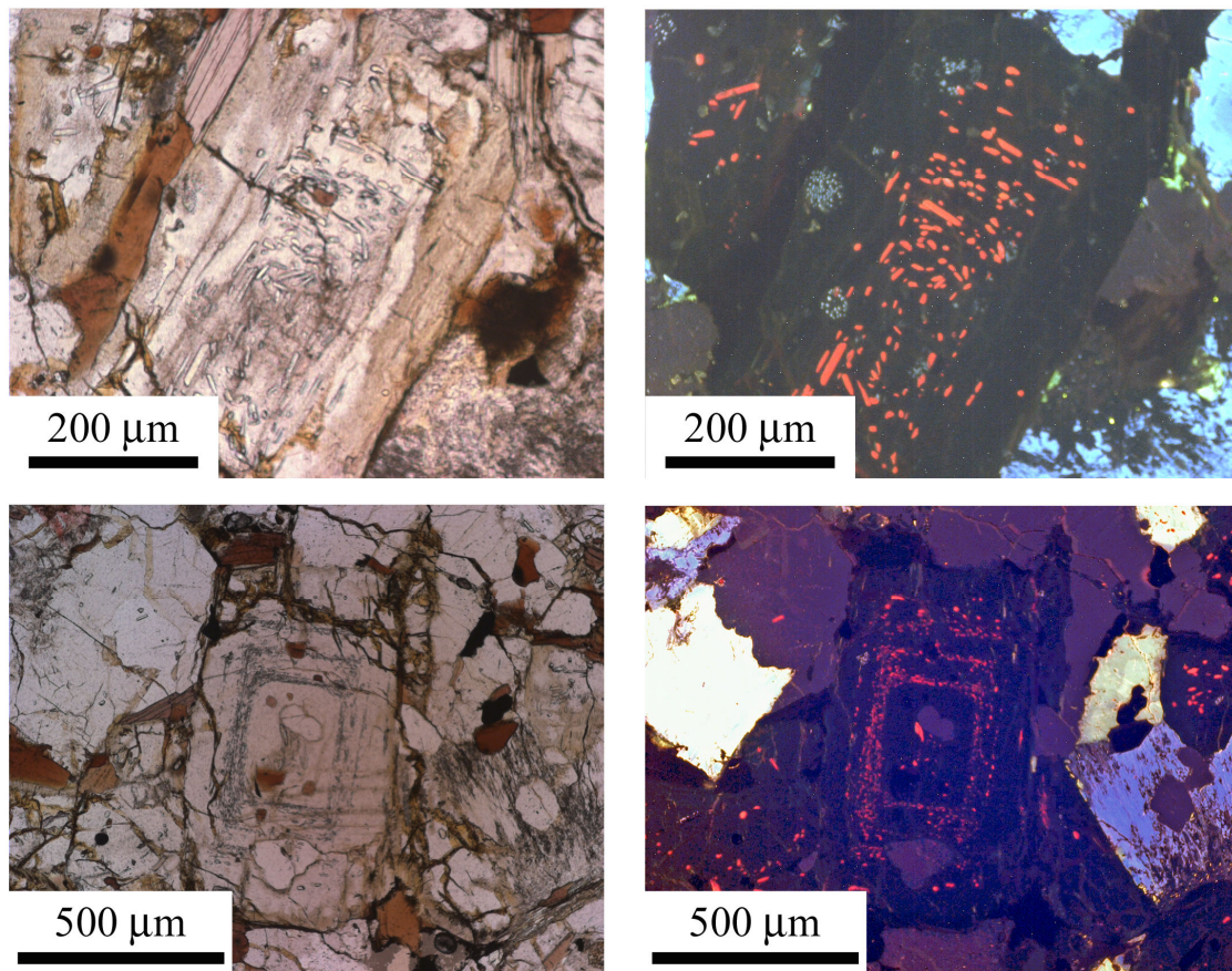
Figure 81 : photos au microscope optique et en cathodoluminescence des cristaux de cordi  rite riches en inclusions
