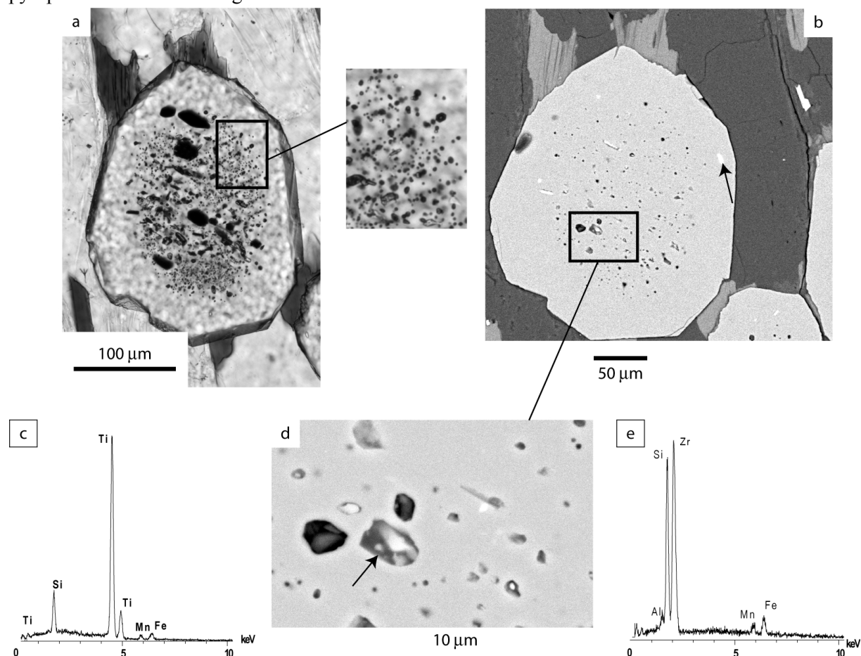
Figure 46 : caractérisation des phases minérales dans un grenat des micaschistes de la série du Chavanon (rutil et zircon)
