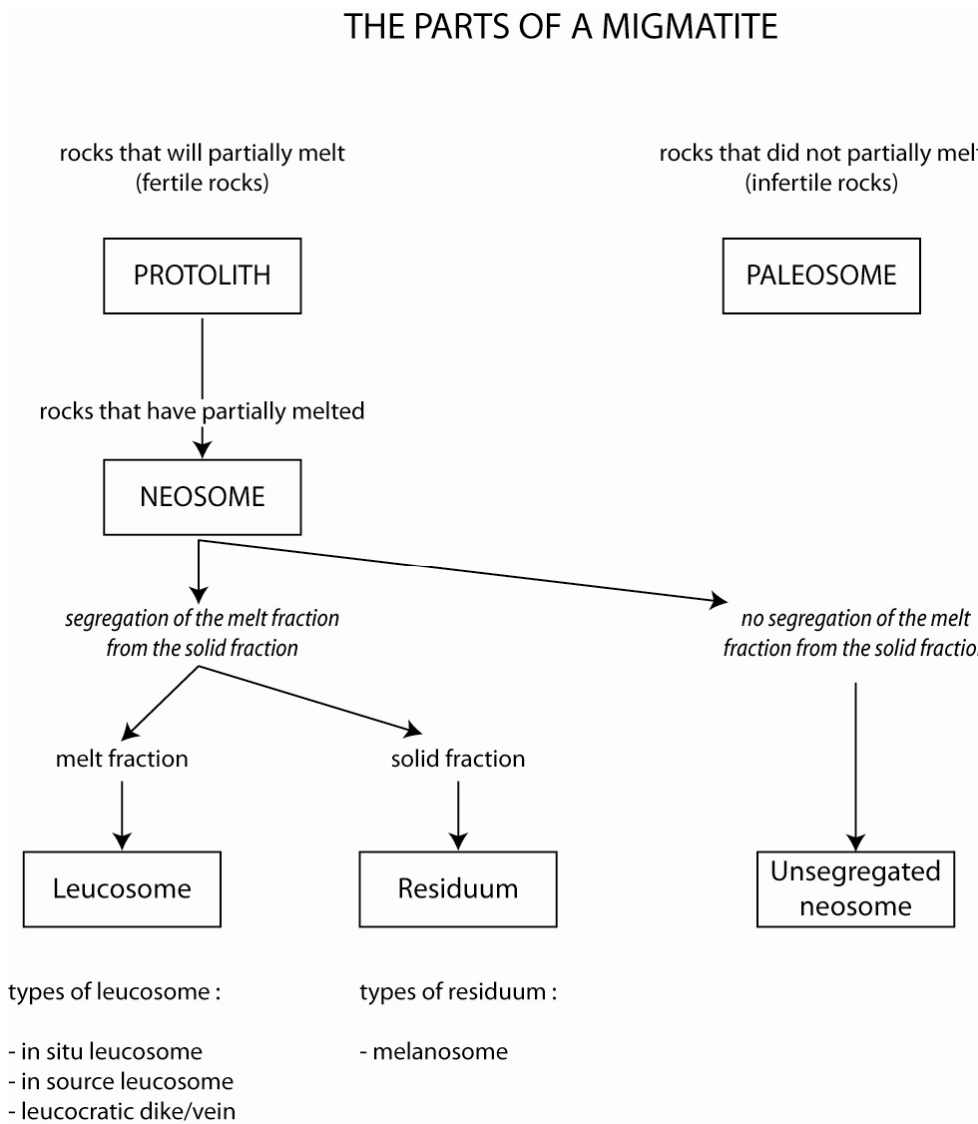
Figure 57 : les différentes parties d'une migmatite selon Sawyer (2008)
