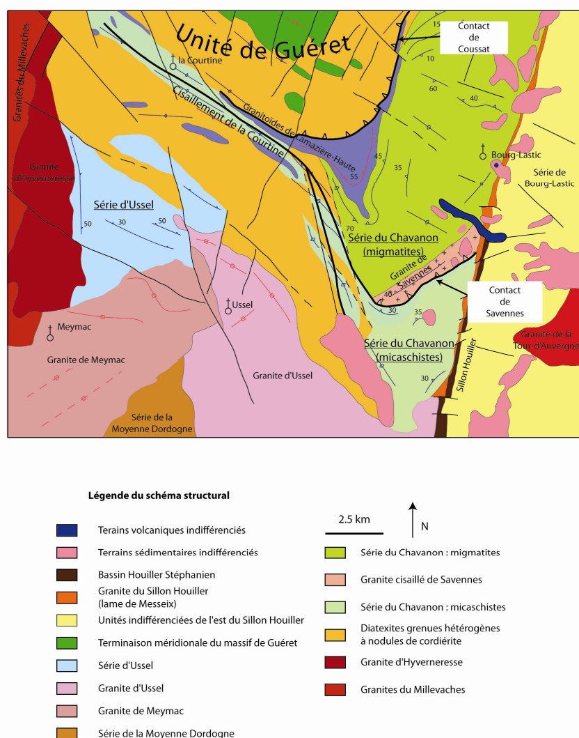
Figure 38 : schéma structural simplifié présentant les unités du Chavanon et d'Ussel dans le cadre de la feuille « Ussel » au 1/50 000
