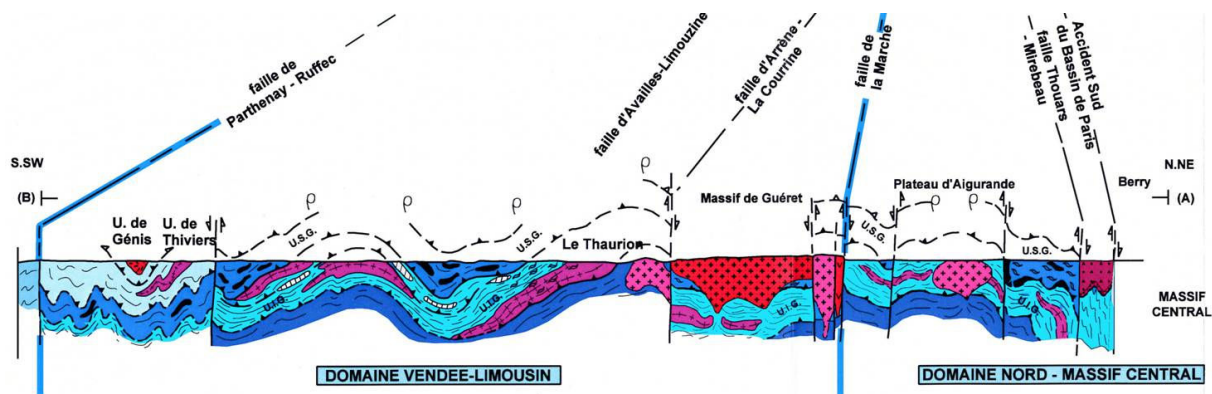
Figure 21 : Coupe à l'échelle crustale montrant la structure en grandes nappes du Massif Central, d'après Rolin & Colchen (2001)
