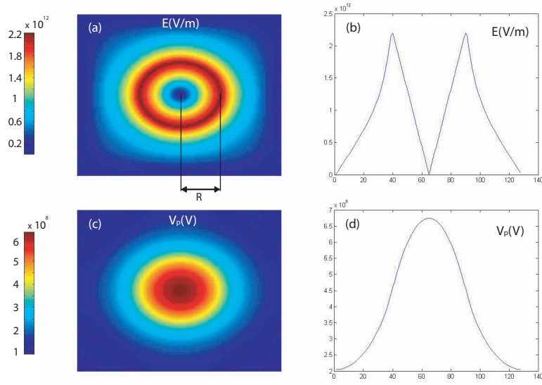
FIGURE 3.17 – Distribution du champ E (a) et du potentiel V (c) et profils du champ (b) et du potentiel (d) selon un diamètre générée pour une sphère uniformément chargée
