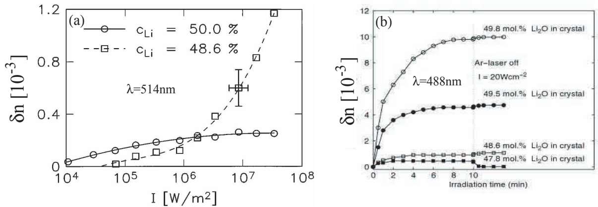
FIGURE 4.3 – Variation de la biréfringence \delta n dans un cristal de LN congruent et stoechiométrique en fonction de l'intensité [168] (a) et l'influence de l'enrichissement en lithium sur la valeur de \delta n en fonction du temps d'exposition à une irradiation lumineuse ( \lambda = 532\text{nm} ) pour I = 10^5 \text{ W/m}^2 (b) [169].
