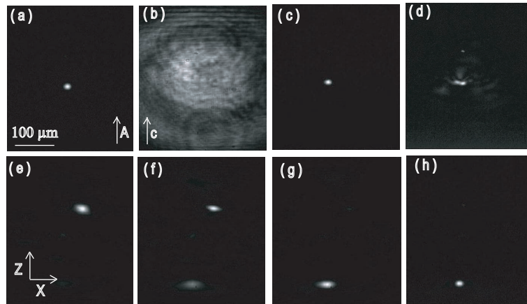
FIGURE 5.5 – Dynamique d'auto-déviation pyroélectriques d'un faisceau laser de polarisation extraordinaire dans un échantillon de LN stoechiométrique. (a) Spot d'entrée, (b) diffraction, (c) maximum de focalisation, (d-f) dynamique de courbure et (e) refocalisation de faisceau.
