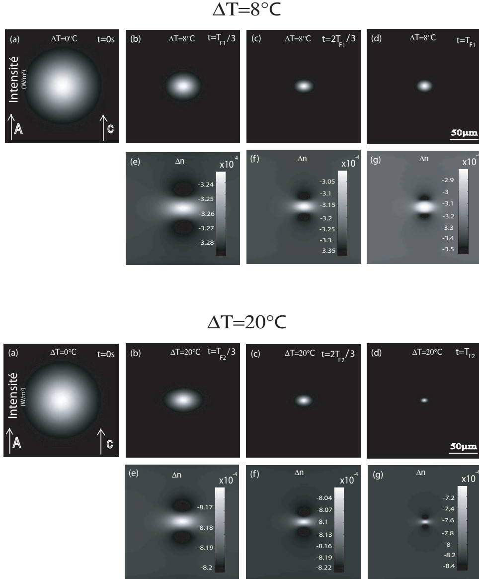
FIGURE 3.21 – Calcul numérique de la dynamique de l'autofocalisation pyroélectrique pour \Delta T = 8^\circ\text{C} et \Delta T = 20^\circ\text{C} dans un échantillon de niobate de lithium de 20\text{mm} de long. Les paramètres de la simulation numérique sont : puissance du faisceau laser 80\mu\text{W} , \Delta T = 8^\circ\text{C} et 20^\circ\text{C} ( \Delta E_{py} = 19\text{KV/cm} et 48\text{KV/cm} ), E_{ph} = 19\text{KV/cm} , N_A = 2 \times 10^{23}\text{cm}^{-3} , N_D/N_A = 2 et I_d = I_{max}/100 .
