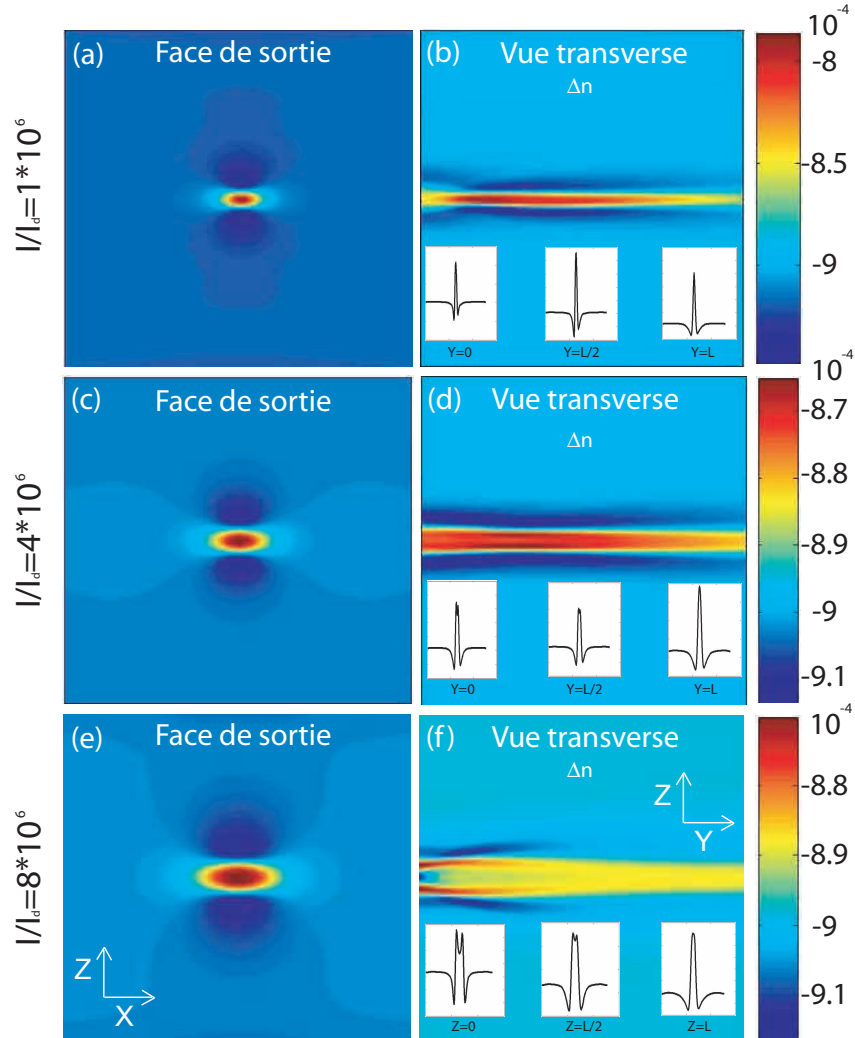
FIGURE 4.24 – Modulations d'indices associés aux spots focalisés des figures 4.23b, d et f respectivement
