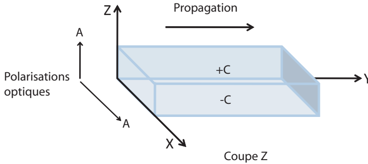
FIGURE 3.2 – Configuration utilisée pour notre étude expérimentale
