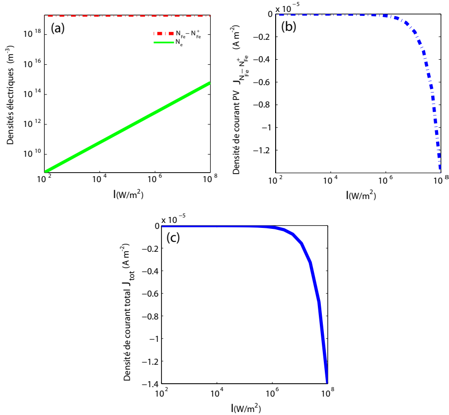
FIGURE 4.20 – Influence de l'intensité lumineuse en régime établi sur la densité de populations du fer (Fe) et des électrons libres (a), du courant photovoltaïque (b) et du courant total (c).
