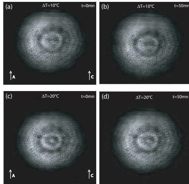
FIGURE 4.15 – Evolution de la diffraction au cours du temps dans le cas d'un court circuit parfait avec une variation de température de 10^\circ\text{C} (a,b) ou 20^\circ\text{C} (c-d).
