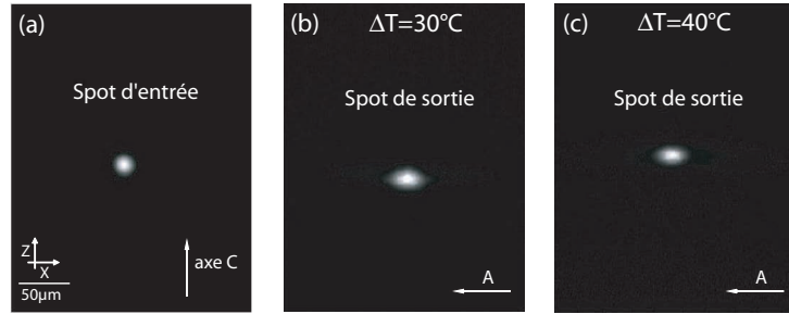
FIGURE 4.11 – Auto-focalisation d'un faisceau de polarisation ordinaire dans un cristal de LN de 17mm de long en fonction de la variation de température. (a) spot d'entrée ( 13\mu m FWHM) (b) focalisation avec une variation de température de \Delta T = 30^\circ C et (c) focalisation avec une variation de température de \Delta T = 40^\circ C . Paramètres : LN congruent X \times Y \times Z = 8mm \times 17mm \times 0.5mm et P = 80\mu W .
