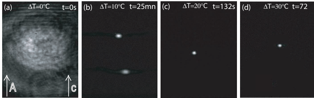
FIGURE 4.5 – Influence de la variation de température sur l'autofocalisation pyroélectriques d'un faisceau laser ( \lambda = 532\text{nm} ) de polarisation extraordinaire dans un échantillon de LN stoechiométrique
