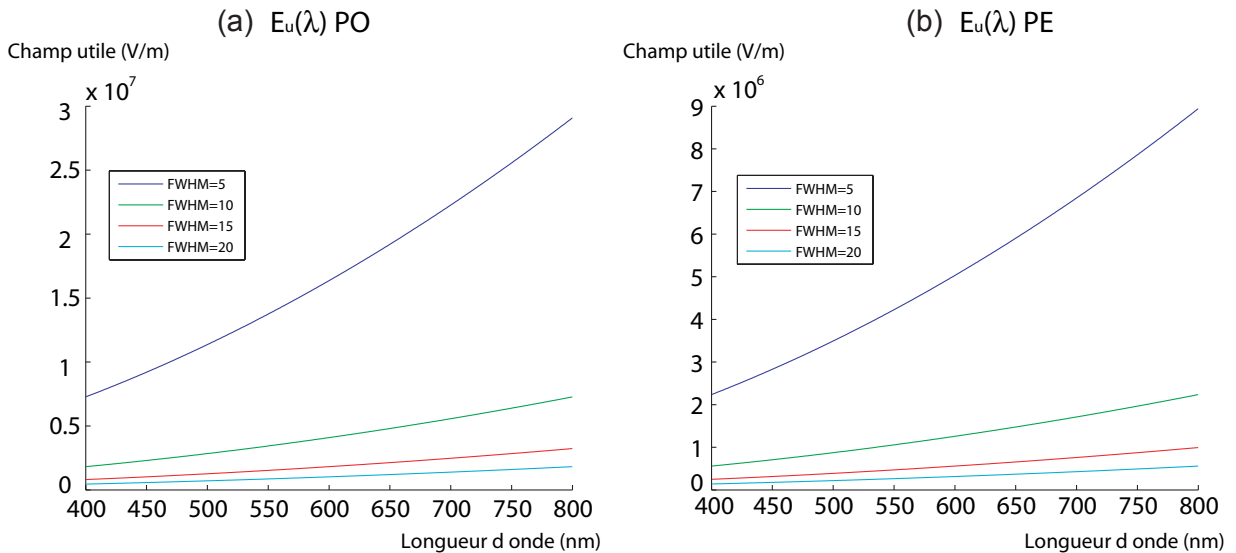
FIGURE 4.38 – Evolution du champ utile E_u pour générer des soliton de taille ( 5\mu m , 10\mu m , 15\mu m et 20\mu m ) en polarisation ordinaire (a) et une polarisation extraordinaire (b) dans le LN en fonction de la longueur d'onde d'induction
