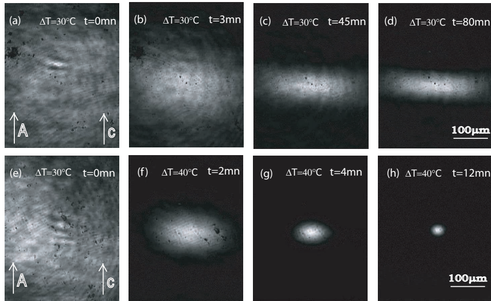
FIGURE 3.6 – Dynamique de l'autofocalisation pyroélectrique dans un échantillon placé 17h à 30°C (a-d) et puis après une augmentation de la température de 10°C (e-h).
