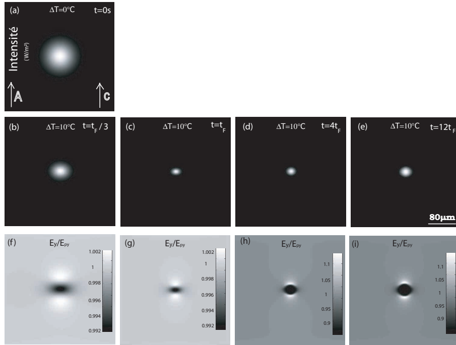
FIGURE 3.20 – Dynamique de l'autofocalisation pyroélectrique (a-e) pour une polarisation extraordinaire dans un échantillon de niobate de lithium de 20mm de long. (f-i) Champ de charge d'espace correspondant aux figures (b-e) respectivement. Paramètres de la simulation numérique : Puissance du faisceau laser 80\mu W , \Delta T = 10^\circ C ( \Delta E_{py} = 24KV/cm ), E_{ph} = 21kV/cm , N_A = 2 \times 10^{23}cm^{-3} , N_D/N_A = 2 et I_d = I_{em}/100 .
