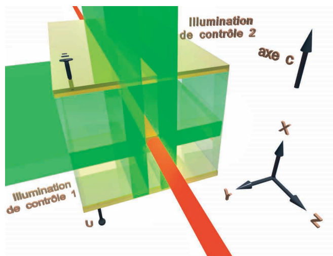
FIGURE 1.16 – Schéma de photo-inscription de guides 2-D dynamiques et reconfigurables utilisant l'illumination latérale. Eclairage de contrôle (faisceaux verts) et faisceau sonde (faisceau rouge) [108].
