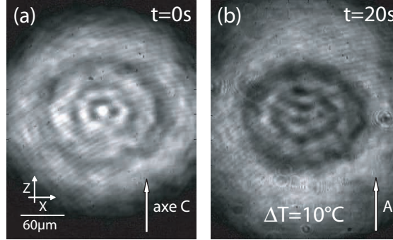
FIGURE 4.16 – Evolution de la diffraction au cours du temps dans le cas d'un court circuit parfait avec une variation de température de 10^\circ\text{C} . (a) Diffraction pour I \approx 10^3 \text{W/m}^2 et (b) défocalisation pour I \approx 10^6 \text{W/m}^2
