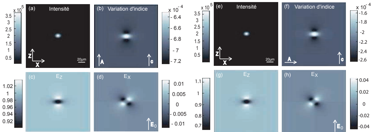
FIGURE 4.34 – Résultats numériques d'un soliton brillant 2D de 15μm à FWHM induit en polarisation extraordinaire (figure de gauche) et en polarisation ordinaire (figure de droite). Images en sortie en régime établie de distribution d'intensité (a, e), variation d'indice \Delta n (b, f), composante du champ de charge d'espace selon l'axe Z(C) (c, g) et composante du champ de charge d'espace selon l'axe X.
