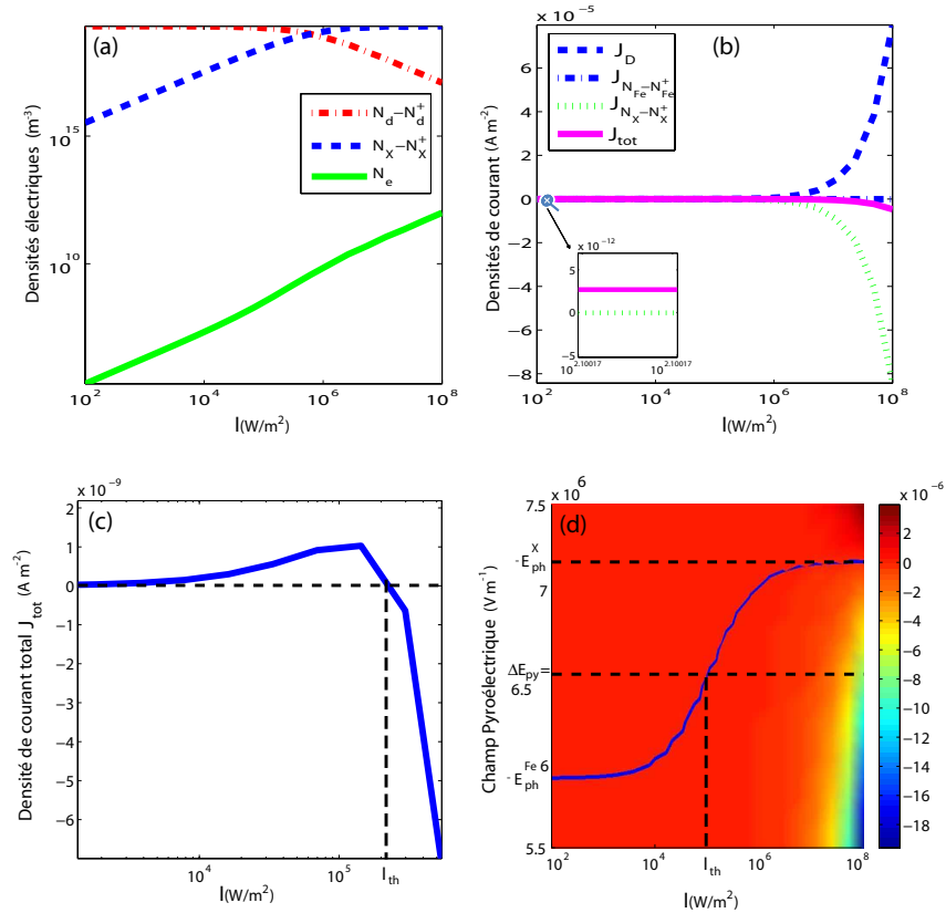
FIGURE 4.22 – (Densité de population de polarons, fer (Fe) et d'électrons libres (a), courants photovoltaïque, d'entraînement et de courant total (b) et densité totale du courant (c) en fonction de l'intensité en régime établie pour E_{py} = 6.5 \times 10^6 V/m . Densité total de courant en fonction de l'intensité et du champ pyroélectrique (d). La courbe de la figure d indique la compensation exacte entre les courants PV et le courant d'entraînement.
