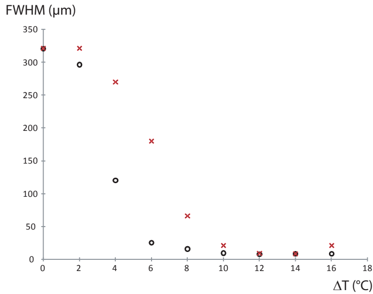
FIGURE 3.15 – Evolution de la taille minimale atteinte en fonction de \Delta T , "○" taille selon l'axe C et "×" taille selon l'axe perpendiculaire à C.
