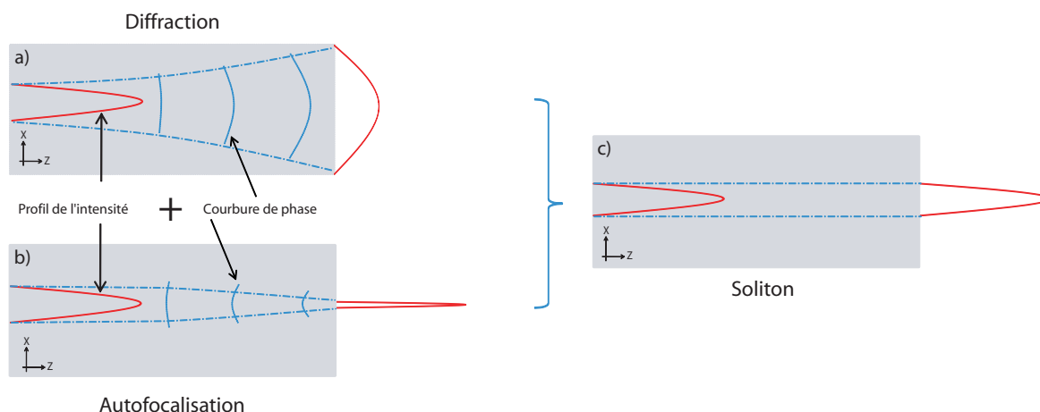
FIGURE 1.4 – Schéma descriptif de la formation d'un soliton spatial.
