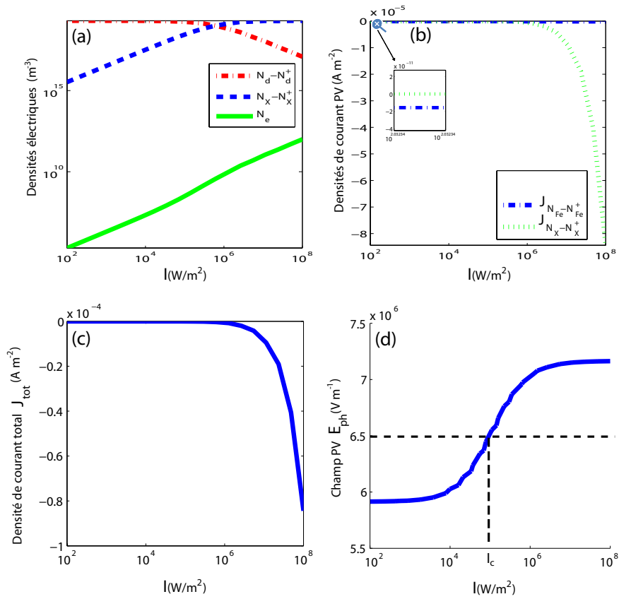
FIGURE 4.21 – Densité de population des polarons, du fer (Fe) et des électrons libres (a), du courant photovoltaïque (b) et du courant total (c) et évolution du champ photovoltaïque (d) en fonction de l'intensité en régime établi.
