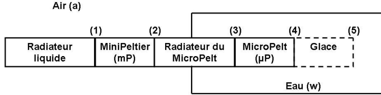
FIG. 4.1 – Structure du micromanipulateur immergé par changement de phase modélisé par analogie électrique.
