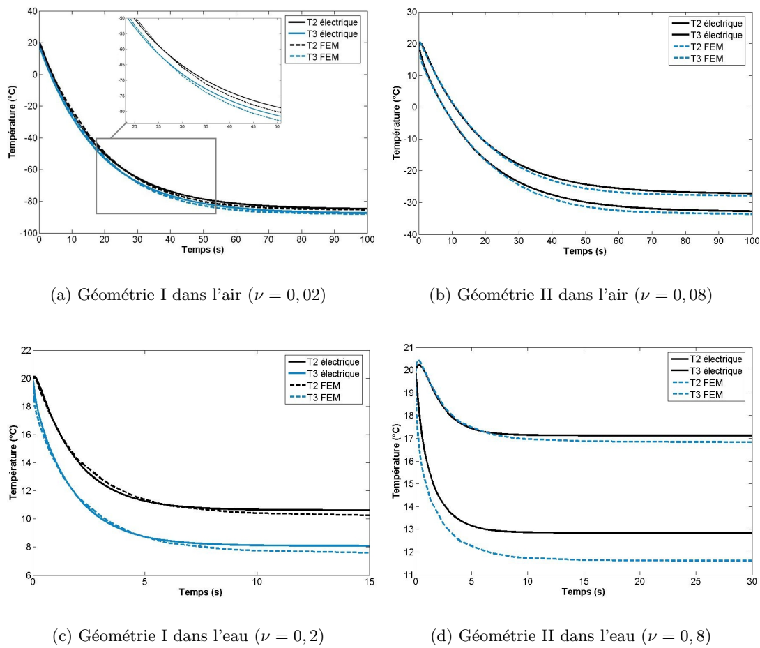
FIG. 3.13 – Températures T_2 et T_3 pour deux géométries testées dans l'air et dans l'eau.
