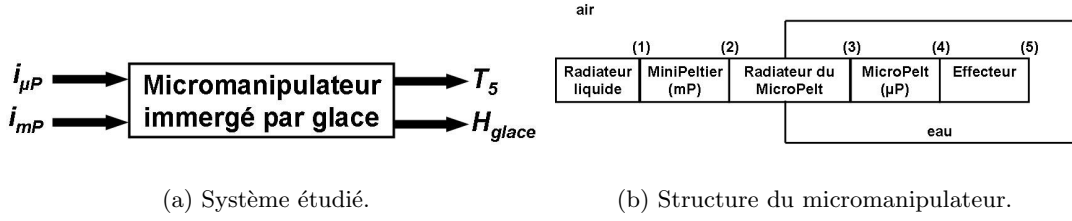
FIG. 2.16 – Schématisation du système de micromanipulation immergée par changement de phase.
