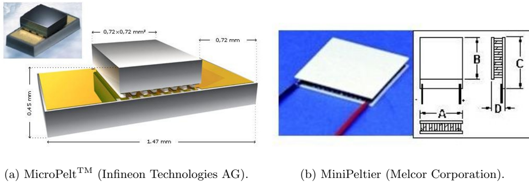
FIG. 2.15 – Modules à effet Peltier utilisés dans le micromanipulateur immergé par changement de phase.
