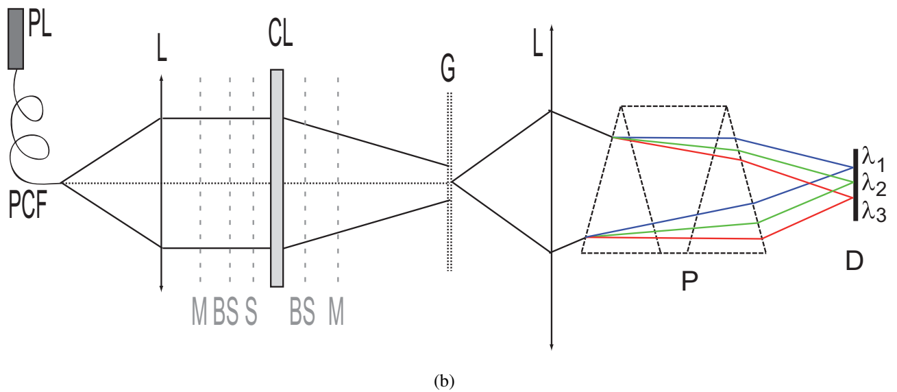
FIG. 2.22 – (a) Schéma représentatif du dispositif SOCT. PL : pompe laser ; M : miroirs ; S : échantillon ; O : objectifs de microscope (NA 0,1 ou 0,25) ; BS : cubes séparateurs polarisés ; QW : lames quart d'onde ; HW : lames demi onde ; CL : lentille cylindrique ; G : réseau de diffraction en transmission 528traits/mm ; L : lentille (focale de 100mm) ; P : Prisme ; D : détecteur CCD. (b) Schéma du démultiplexage en longueur d'onde via le prisme, la lentille cylindrique est insérée à la sortie de l'interféromètre de Linnik.
