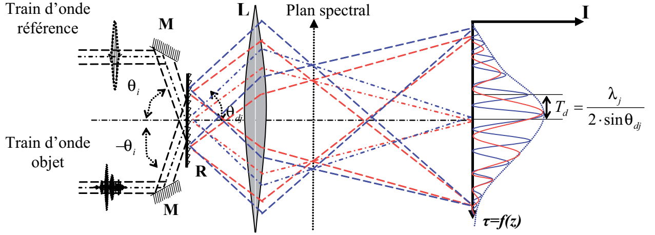
FIG. 2.10 – Échantillonnage du signal d'interférence par un réseau de diffraction par transmission.
