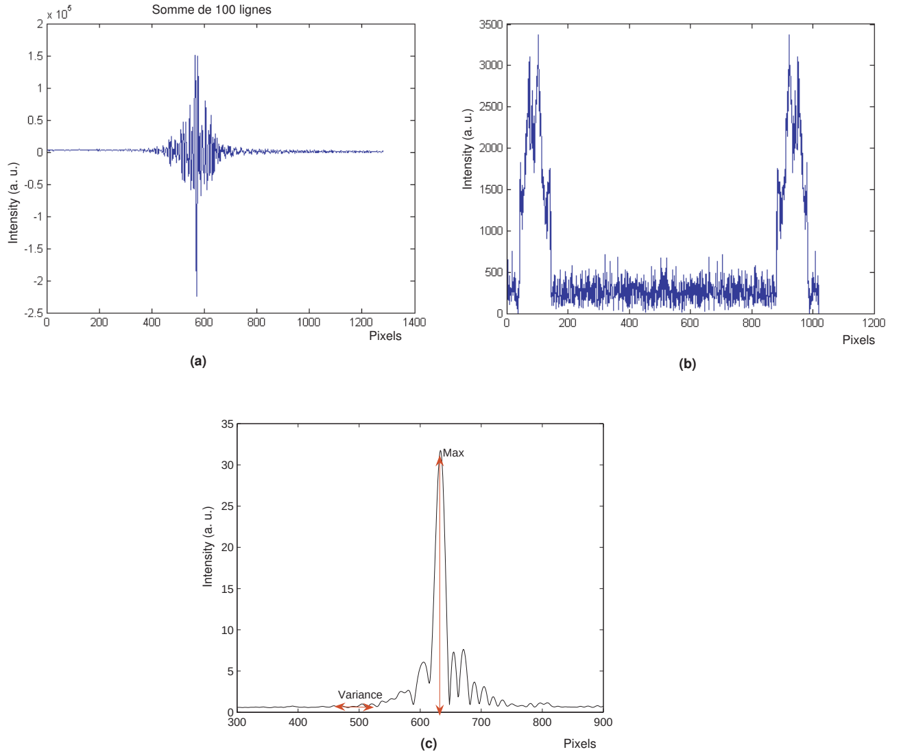
FIG. 3.10 – (a) Signal d'interférence sans DC. (b) transformée de Fourier du signal d'interférence. (c) Module de la transformée de Fourier inverse après filtrage.
