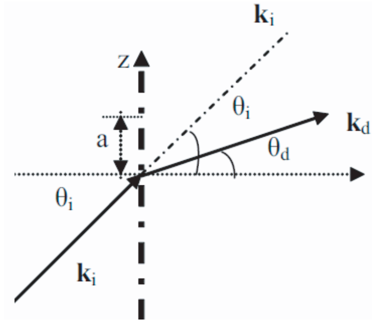
FIG. 2.8 – La relation fondamentale des réseaux sous forme vectorielle.
