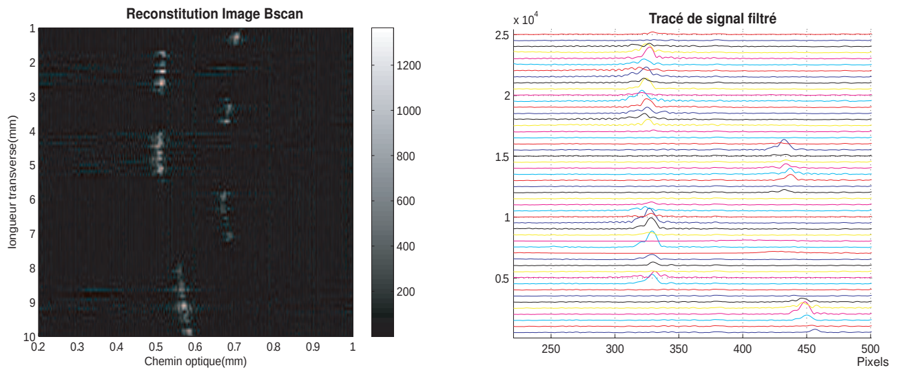
FIG. 3.15 – Une image 2D et quelques profils de réflectivité A-scan d'une ligne de la pièce de 50 centimes indiquée par le trait horizontal montré sur la figure 3.14. (a) Affichage d'une image B-scan (XZ) obtenue en post-traitement de la ligne de la pièce de 50 centimes. Les trois tâches blanches situées à la profondeur entre 0,65mm et 0,75mm correspondent à la lumière réfléchiée par la surface du motif et les trois spots localisés à la profondeur entre 0,52mm et 0,58mm coïncident avec la lumière issue de la surface de la pièce. (b) Un tracé de quelques acquisitions A-scan filtrées correspondantes à la ligne X de la pièce de 50 centimes englobées dans une matrice (i, j) .
