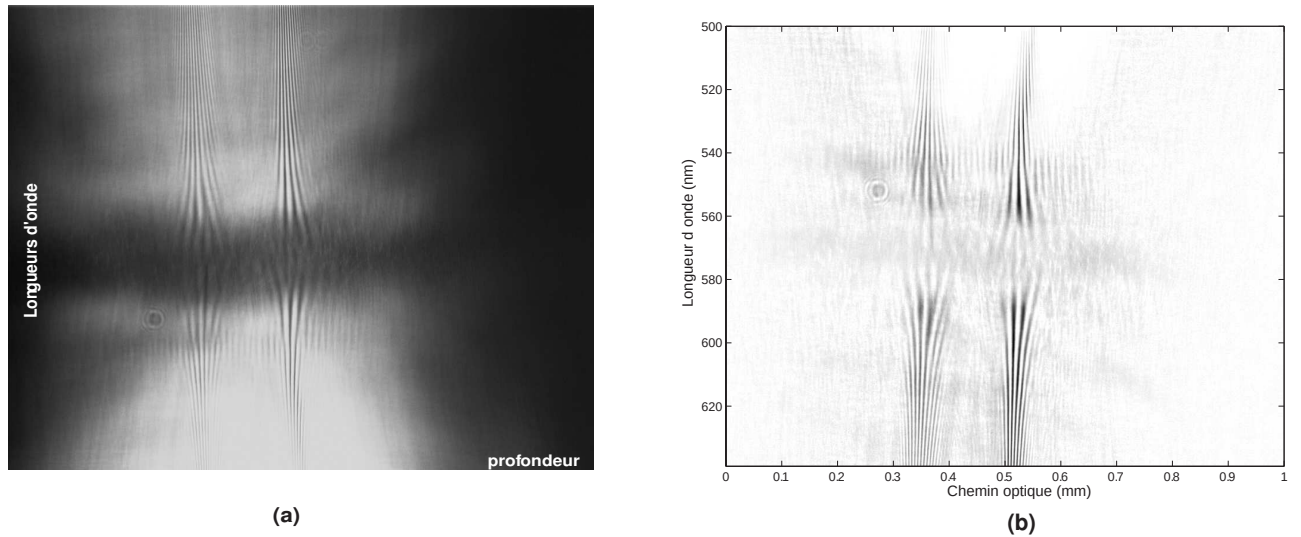
FIG. 3.20 – Spectro-corrélation d'une lame de verre. (a) Image brute. (b) Image traitée avec le logiciel Image J.
