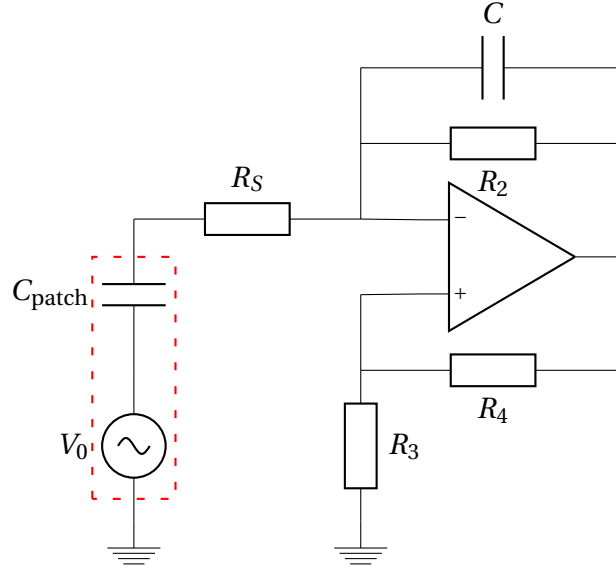
FIG. 3.1: Réalisation d'un circuit analogique à capacité négative à partir d'amplificateurs opérationnels.
