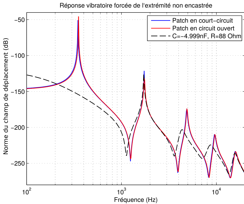
FIG. 4.7: Réponse vibratoire forcée de l'extrémité non encastrée.
