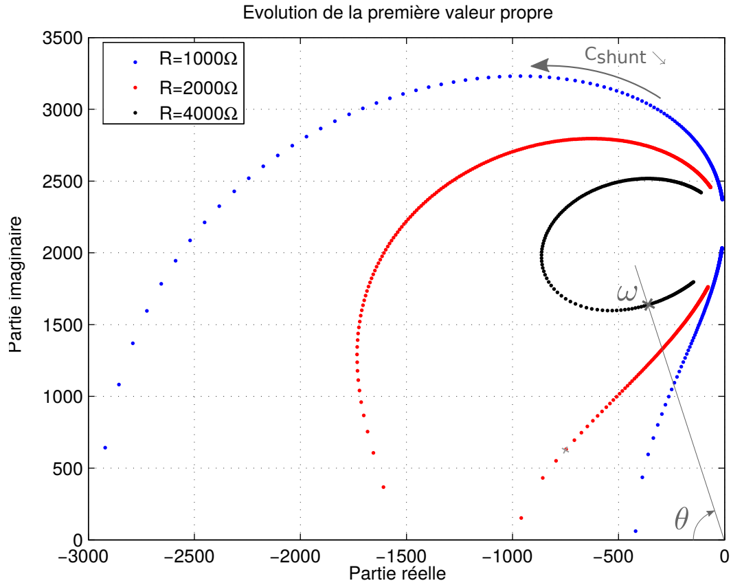
FIG. 4.14: Évolution de la première valeur propre en fonction de la capacité du shunt.
