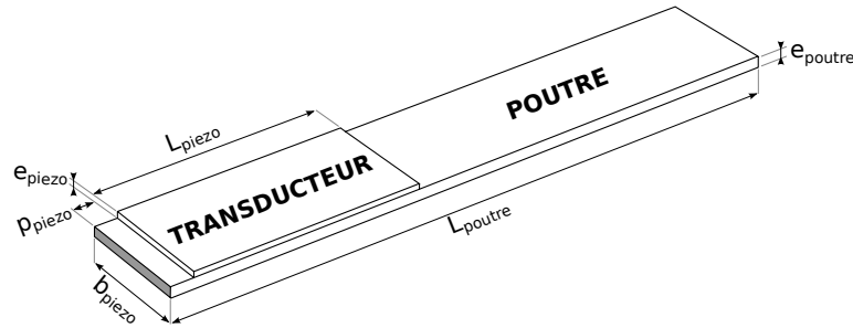
FIG. 4.2: Système étudié.
