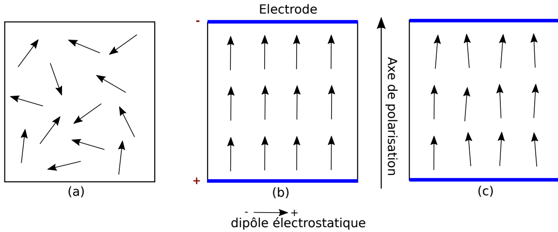
FIG. 2.2: Processus de polarisation [36]: (a) dipôles orientés aléatoirement avant la polarisation; (b) un fort champ électrique continu est appliqué; (c) il reste une polarisation rémanente après la disparition du champ.
