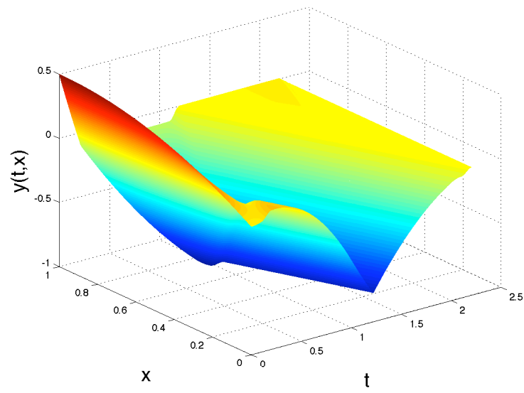
FIG. 1.31: Solution contrôlée y_\epsilon dans (0, T) \times (0, 1) .
