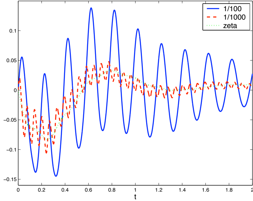
FIG. 1.20: T = 2, k = 1/5, \alpha = \mathbf{0} , u^\varepsilon(\cdot, L) pour \varepsilon = 10^{-2} (ligne pleine), \varepsilon = 10^{-3} (ligne tiretée) et la limite \zeta (ligne pointillée) vs. t \in [0, T] .
