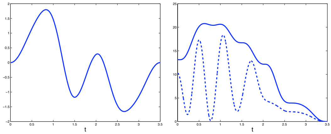
FIG. 1.26: Gauche : contrôle v(t) vs. t \in (0, T) ; Droite : Energie (ligne pleine) et énergie cinétique (ligne tiretée) vs. t \in (0, T) .
