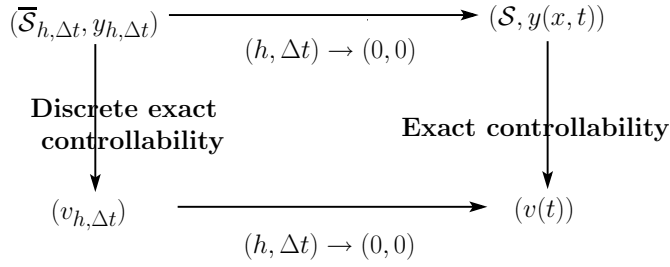
FIG. 1.2: Diagramme de commutativité associé au schéma modifié (\bar{S}_{h,\Delta t}) pour \Delta t < h\sqrt{T/2} .
