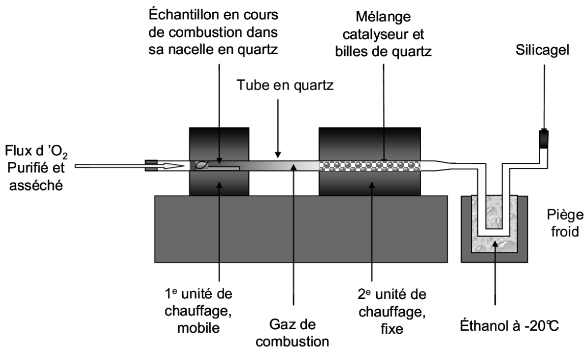
Figure 2-1 : Représentation schématique du dispositif d'extraction du tritium organiquement lié (Boyer, 2009)
