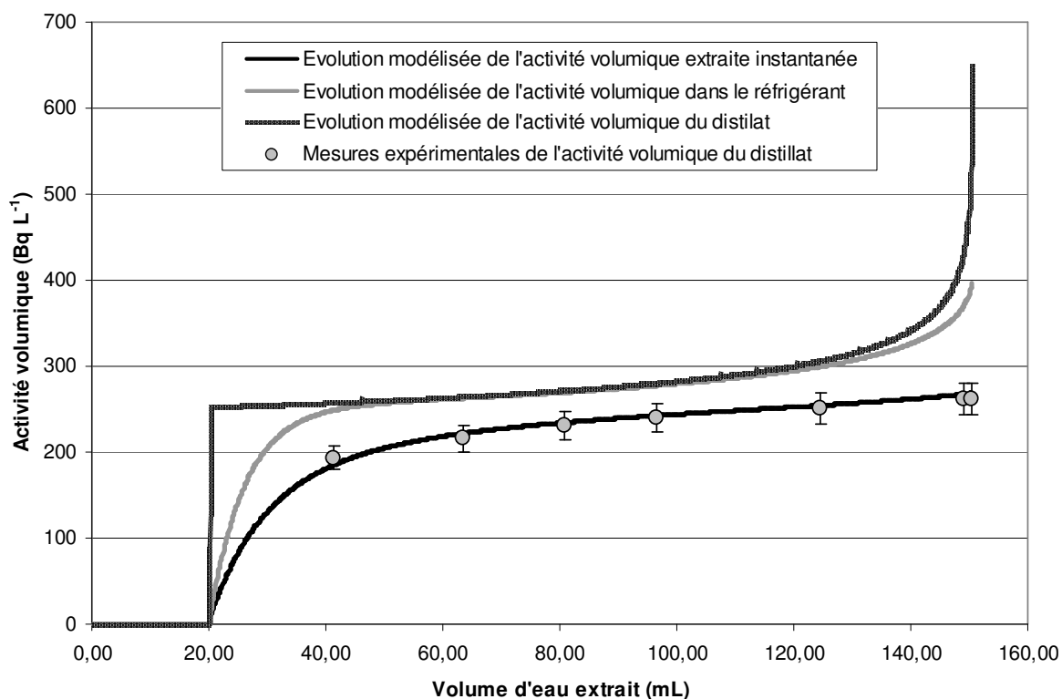
Figure 3-12 : Modélisation de l'évolution de l'activité volumique extraite instantanée et des activités volumiques de l'eau dans le réfrigérant et le distillat d'un évaporateur rotatif Les vingt premiers millilitres correspondent à la saturation préalable du volume mort du réfrigérant en eau non-tritiée. Les barres d'erreur représentent les incertitudes de mesures.
