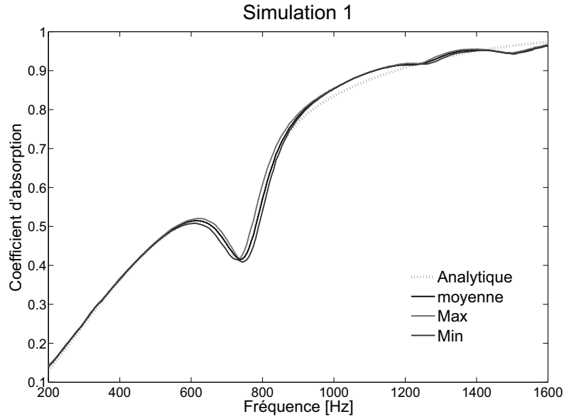
FIG. 4.4: Coefficient d'absorption pour une mousse mélamine (Simulation 1)
