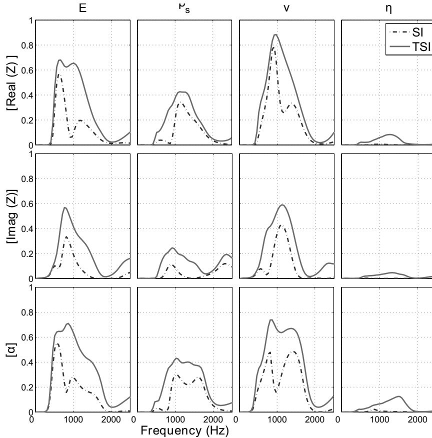
FIG. 4.2: Analyse de la sensibilité des paramètres de mécaniques pour la mousse de mélamine.
