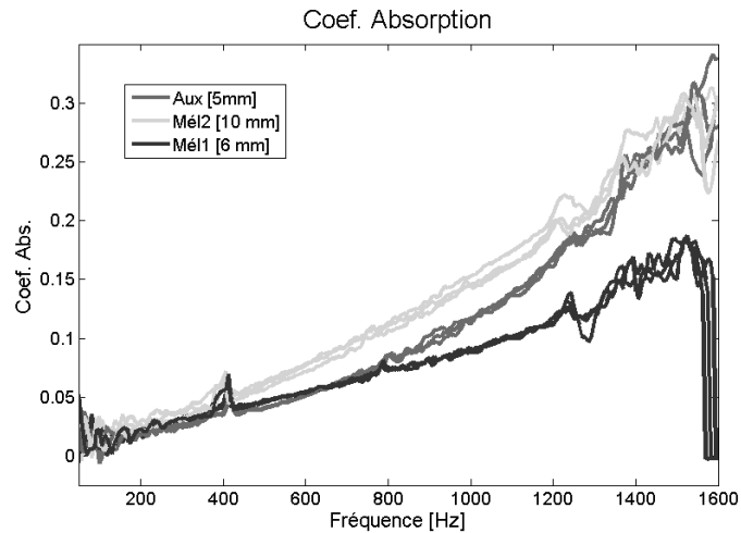
FIG. 5.4: Mesures du coefficient d'absorption dans la bande de fréquence de 50 Hz à 1.6 kHz pour des échantillons de 100 mm de diamètre.
