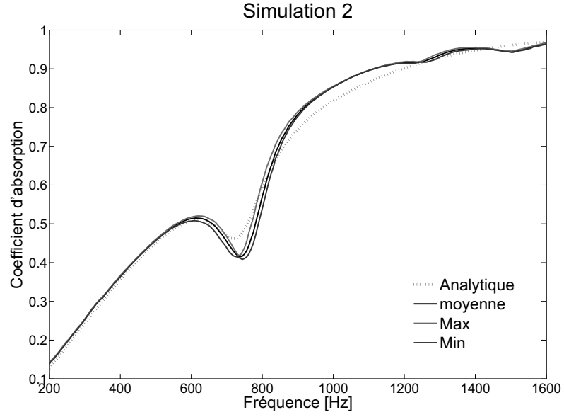
FIG. 4.6: Coefficient d'absorption pour une mousse mélamine (Simulation 2)
