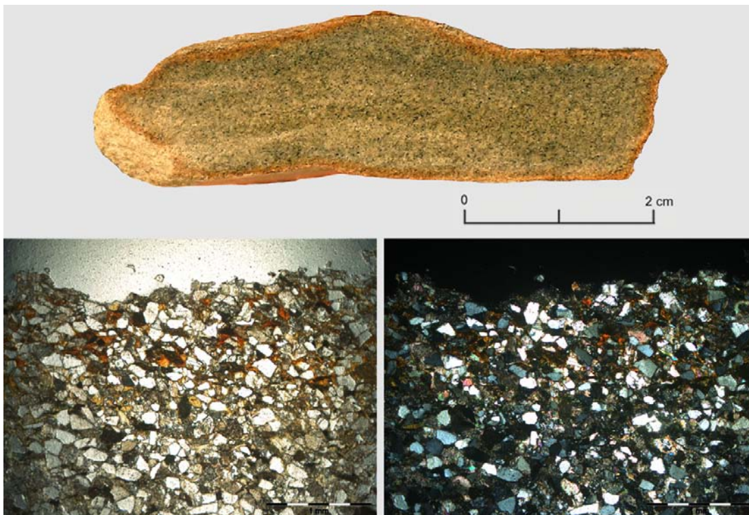
Figure 127 : polissoir de CH 4 phase 4, n° 1442 33, grauwacke calcaire. La chauffe du polissoir se traduit par une rubéfaction de la surface, visible en coupe et en lame mince (LN à gauche, LP à droite), par l'oxydation des minéraux et la transformation d'une partie de la calcite en chaux
