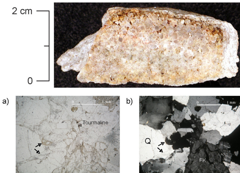
Figure 107 : cliché à l'œil nu, en LN (a) et LP (b) d'une arkose, objet n° 11911 17, CH 19 O. Notez l'altération de surface de l'artefact, ainsi que la présence de quartz nourri (la limite entre grain originel et auréole de nourrissage est indiquée par des flèches) et de feldspath type microcline
