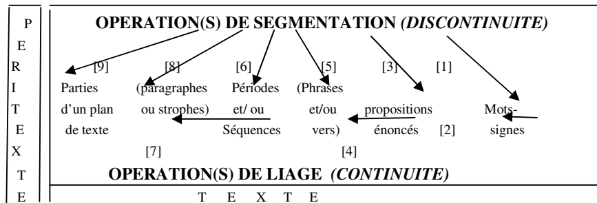
Schéma 4 171 :
