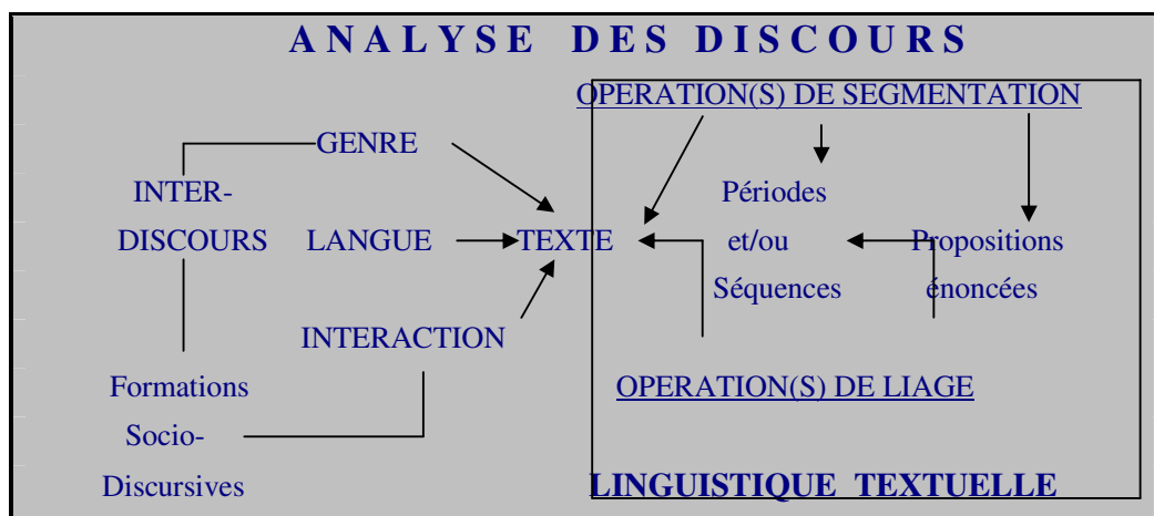
Schéma 2
