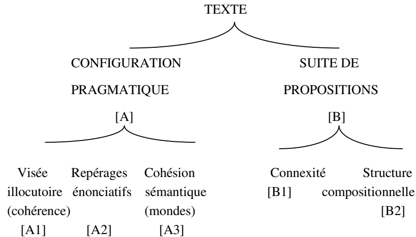
Schéma 1
