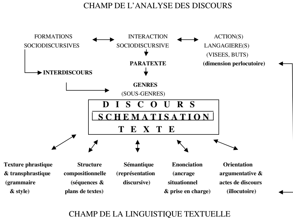
Schéma 3
