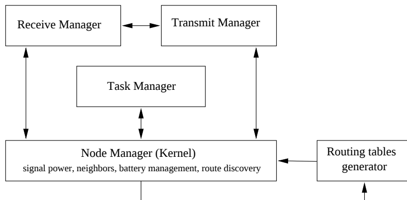
FIG. 7.1 – Les différents composants du simulateur AdhocSim-Net.
