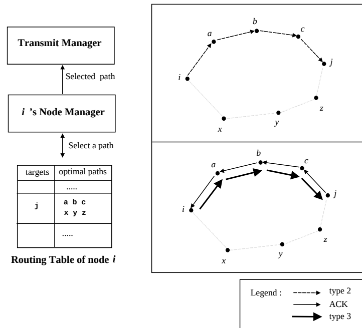
FIG. 7.9 – Routage de données.
