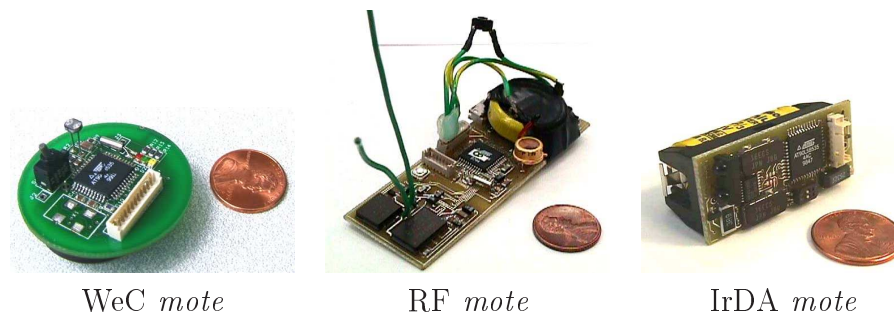
FIG. 3.1 – Quelques nœuds capteurs de type COTS Dust de l'UC Berkeley.
