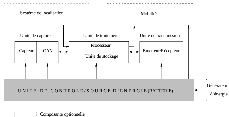
FIG. 1.3 – Architecture d'un nœud capteur
