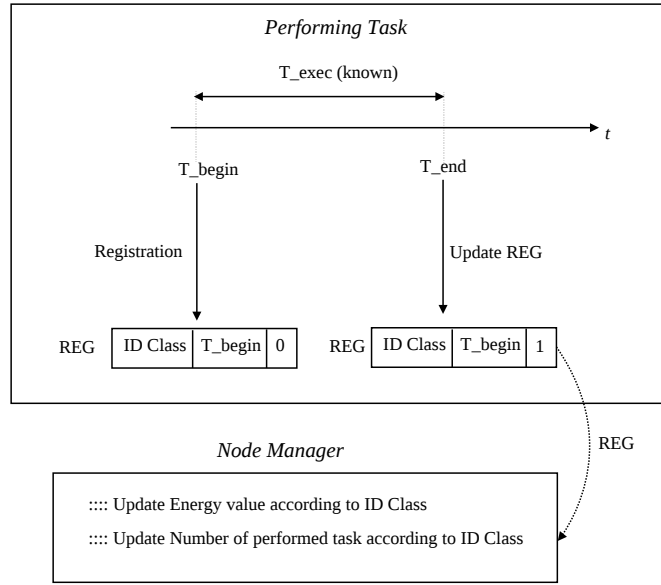
FIG. 7.8 – Simulation de l'exécution d'une tâche.
