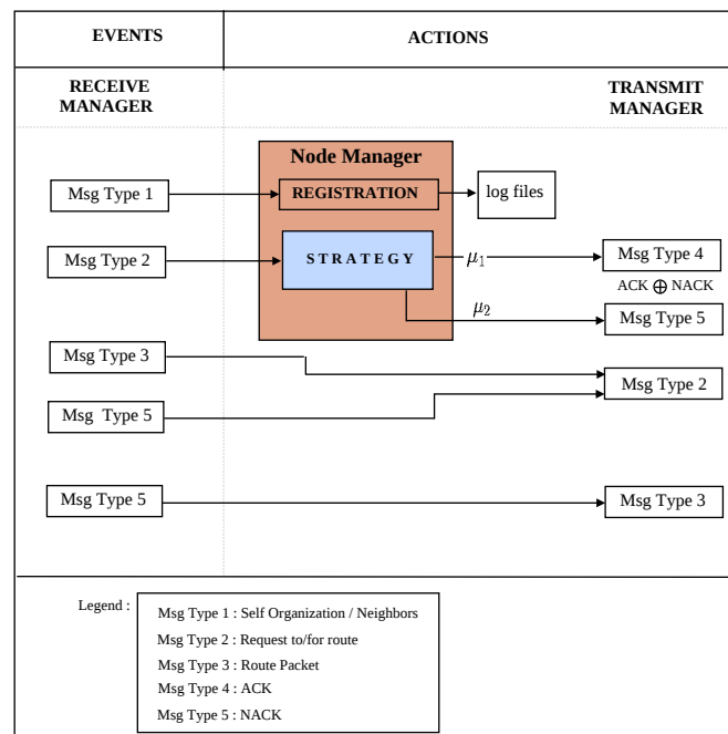
FIG. 7.10 – Gestionnaire de messages.
