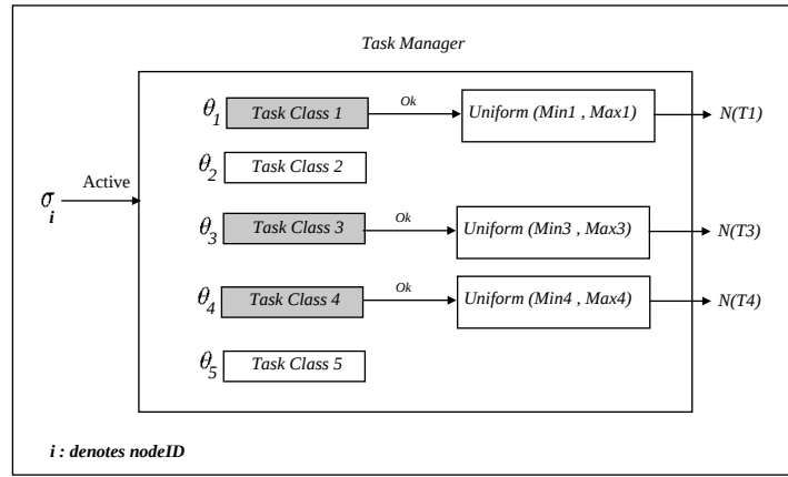
FIG. 7.7 – Gestionnaire de tâches.
