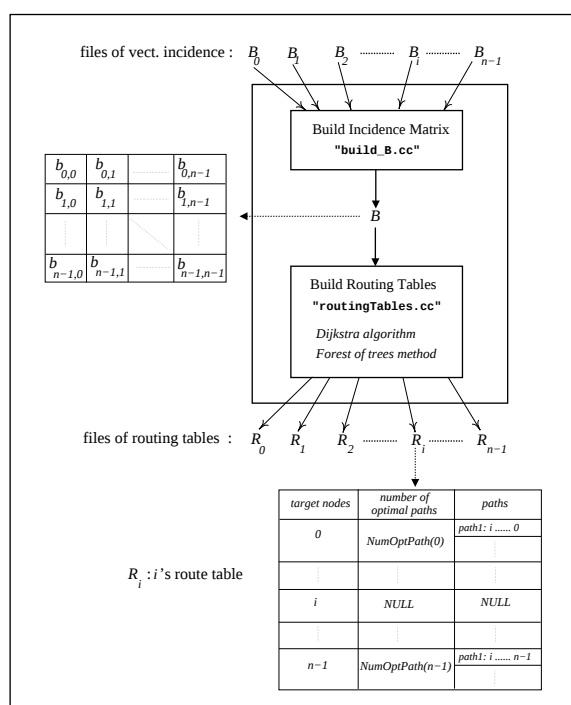
FIG. 7.12 – Génération des tables de routage.
